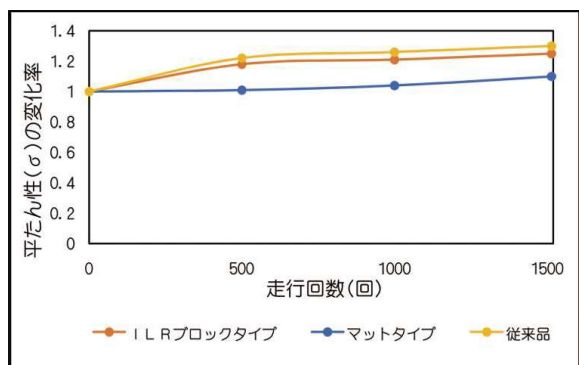
平たん性の変化率と推移
