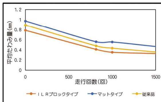
たわみ量の推移
