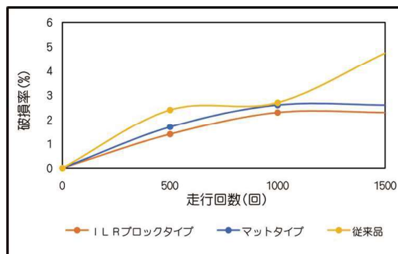
ブロック破損率の推移
